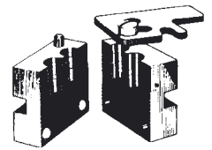
Doppel-Gießkokille
