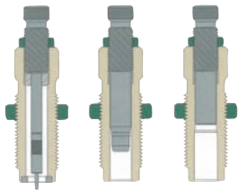
Titanium Carbide Matrizensatz
