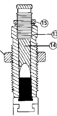
Setzmatrize
