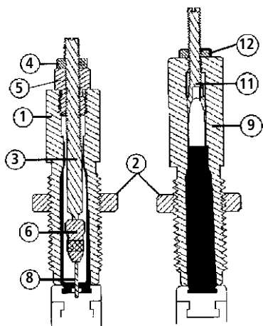
Kalibriermatrize für Büchsenpatronen
