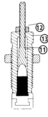
Setzmatrize (alte Ausführung)
