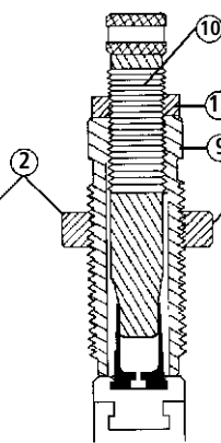
Aufweitematrize für Faustfeuerwaffen
