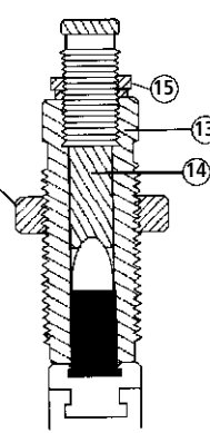
Setzmatrize
